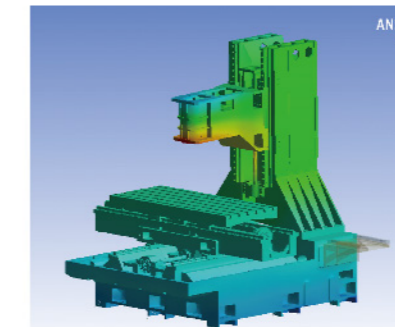
Y AXIS
